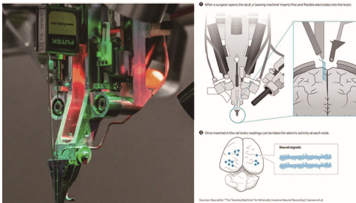
圖四：Neuralink 公司和他們的腦機介面鐳射種植器
