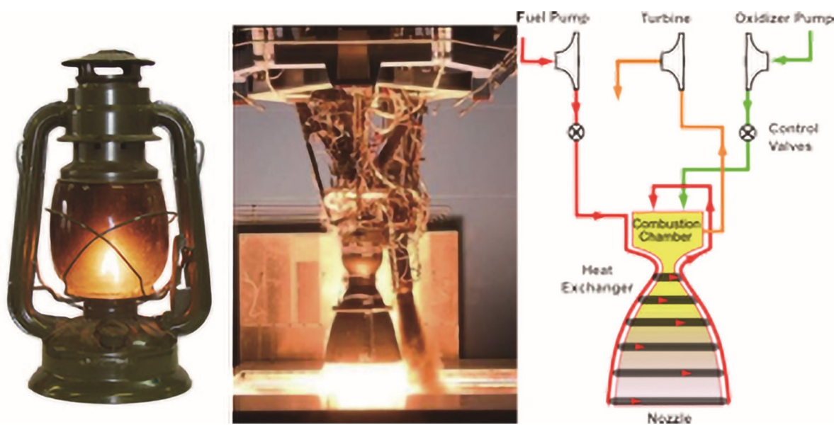
圖三：煤油燈和液氧煤油發動機
